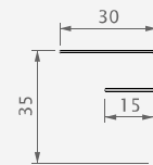
P 105 F-profiel
