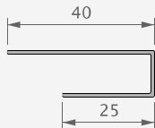
P 109 U-afwerkingsprofiel
